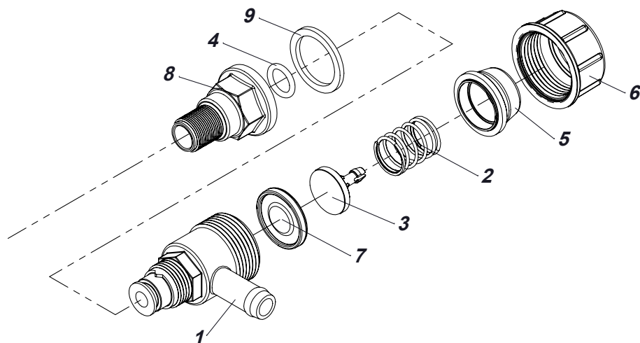
PORTA BICO LATERAL ANTIGOTEJO (17362200)
