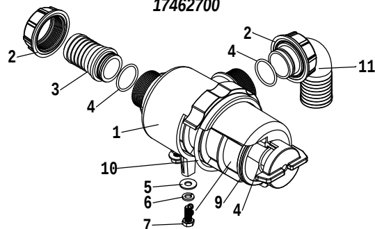
FILTRO DE SUÇÃO 120L C/CONEXÃO 17517400
