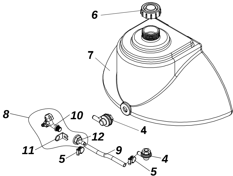
RESERVATORIO DE AGUA LIMPA 20L CPL CÓDIGO: 17337300
