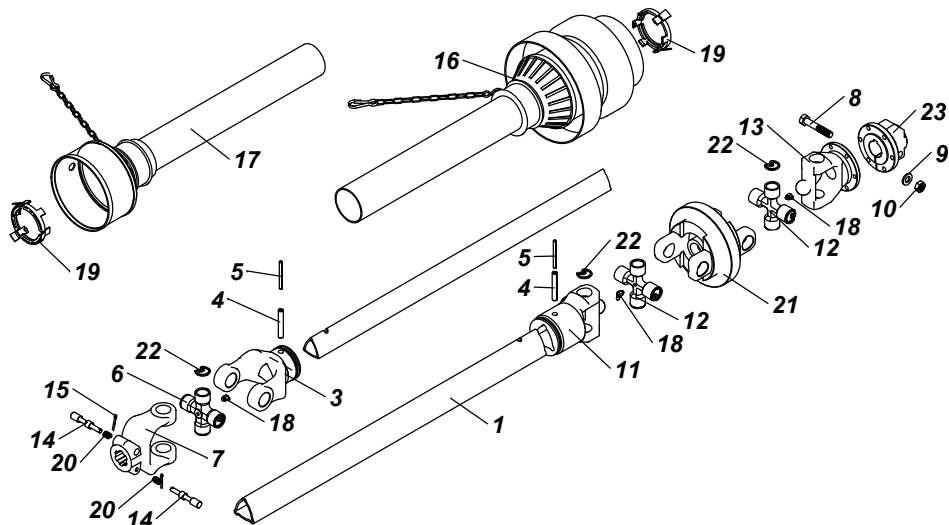
CARDAN HOMOC.SERIE 5000-INVERTIDO Cód: 21140130 EXCLUSIVO PARA CÂMBIO ESTERÇANTE
