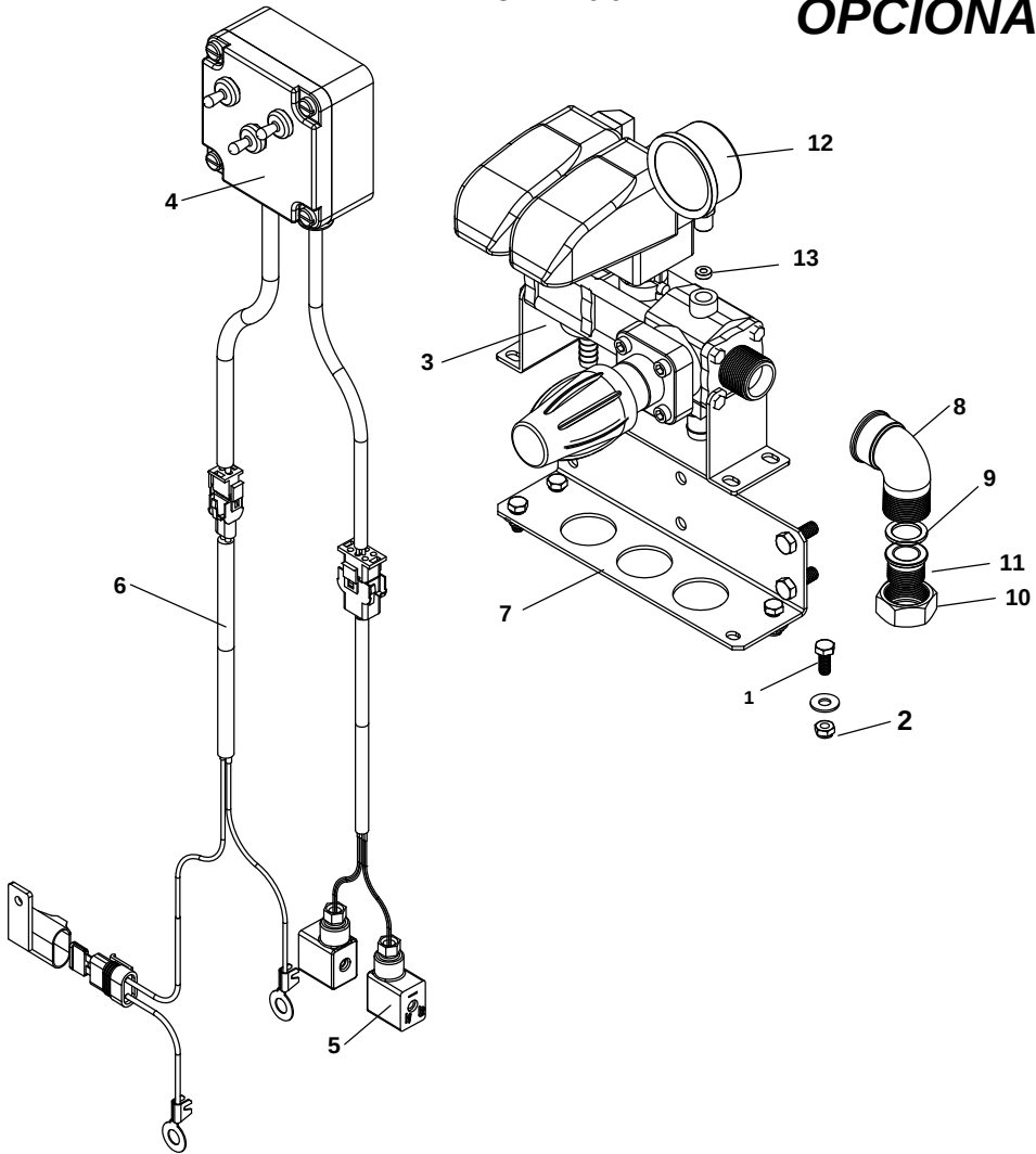
COMANDO GEOLINE
