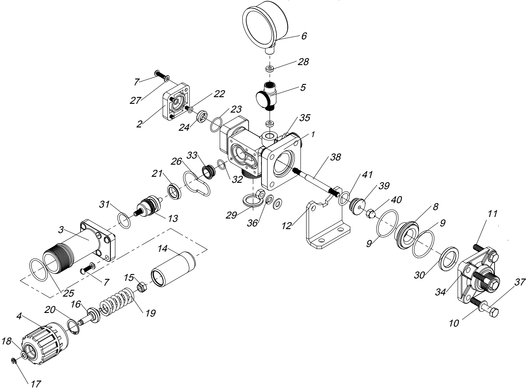
COMANDO - 1 VIA 3PH45 (17213500)
