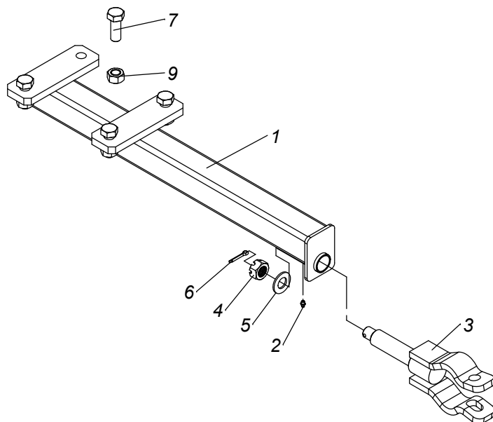
CAMBÃO FIXO KO A500/700/1000 COMPLETO CÓD: 17333900
