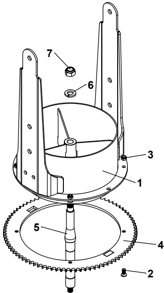
CONDUTOR DIRECIONADOR C/ACIONAMENTO HIDRAULICO COM COROA CÓD: 17395700
