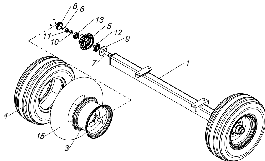
RODEIRO KO A2000 (PNEU 11L-15) -17198000
